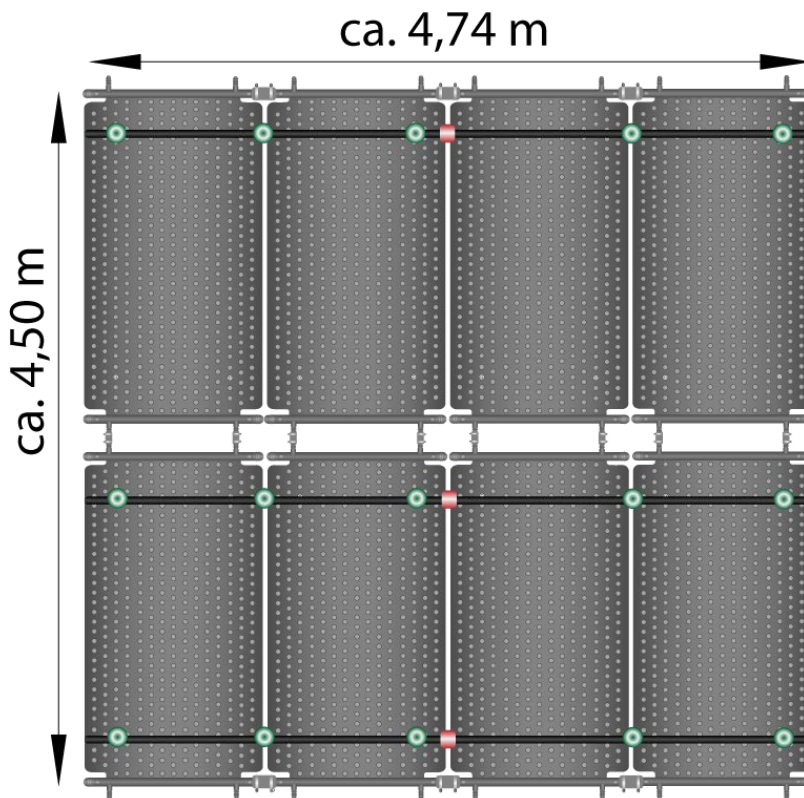
2 Reihen à 4 Absorber senkrecht
