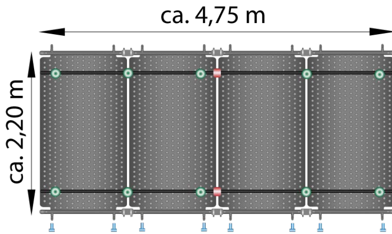
1 Reihe à 4 Absorber senkrecht
